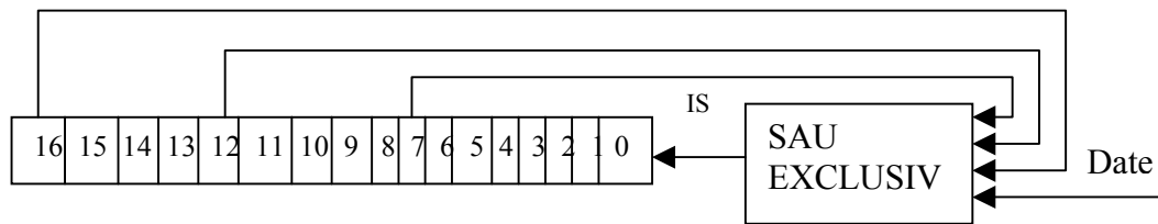
Figura 9.8: Implementarea comprimării
