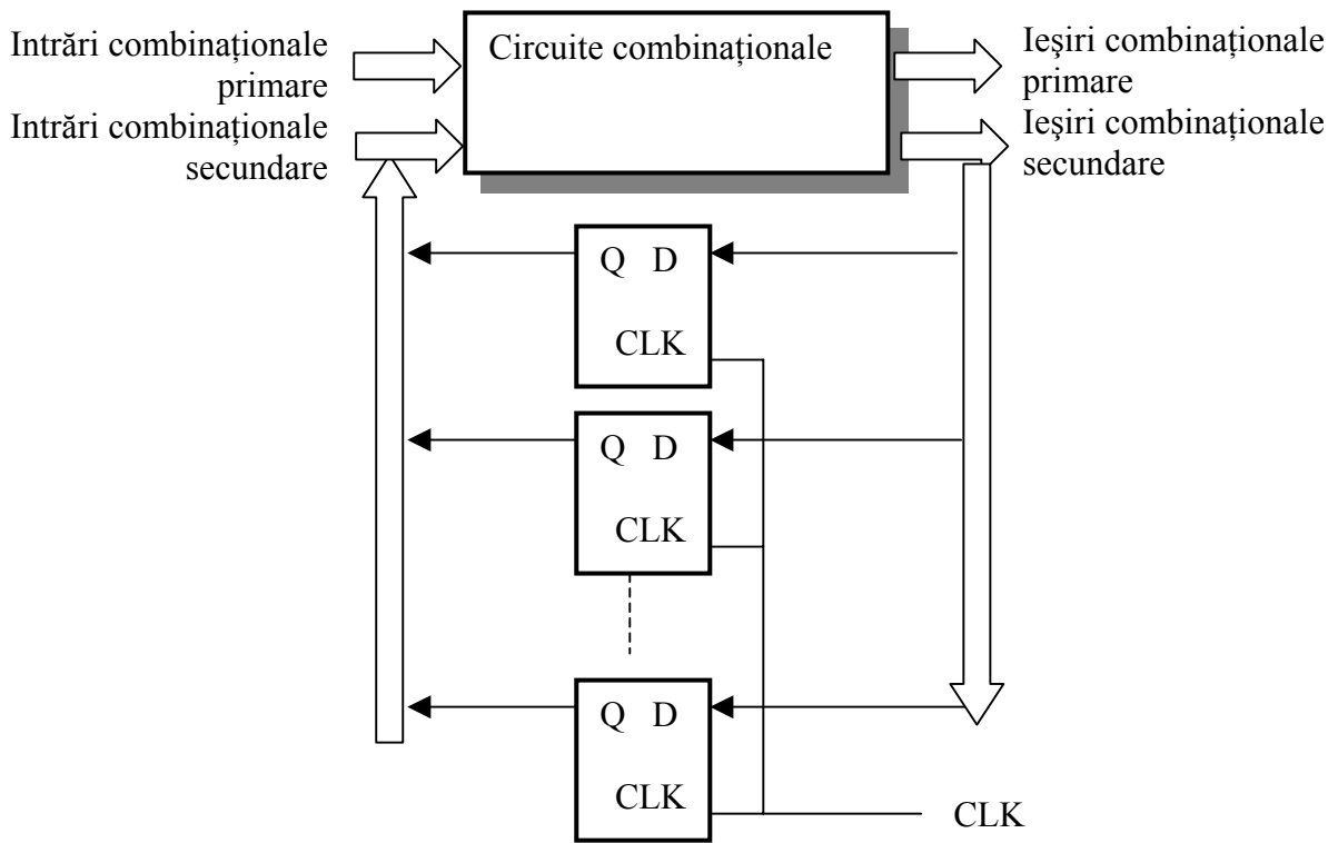
Figura 9.9: Partiționarea unei scheme
