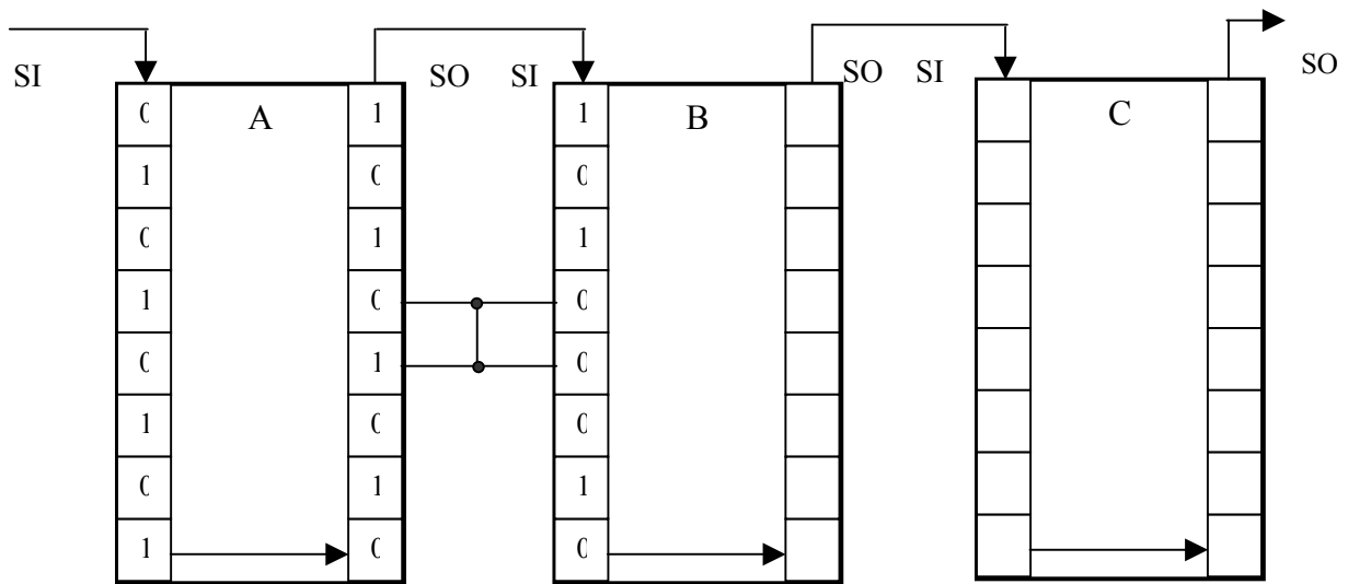
Figura 9.12: Testarea interconexiunilor
