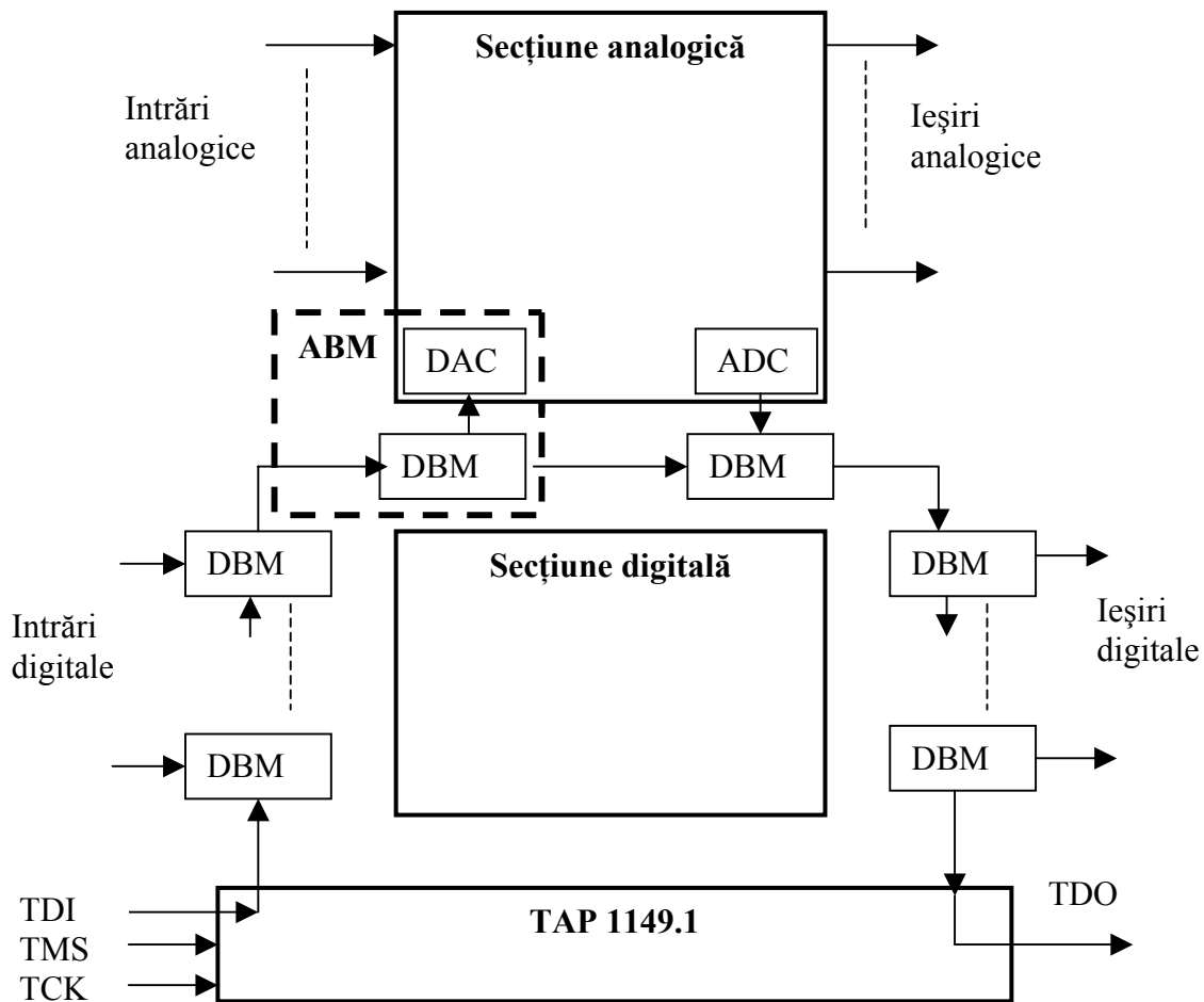
Figura 9.14: Structura de testare analogică și digitală
