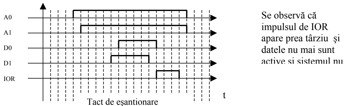
Figura 9.5: Afișarea datelor la un analizor logic
