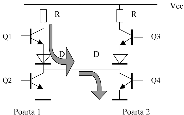
Figura 9.3: Scurtcircuit între două trasee de semnal
