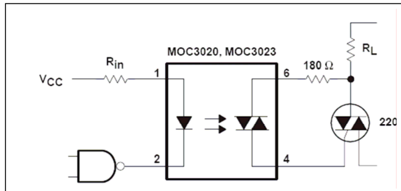
Figura 6.3: Comanda digitală a triacului cu optotriac
