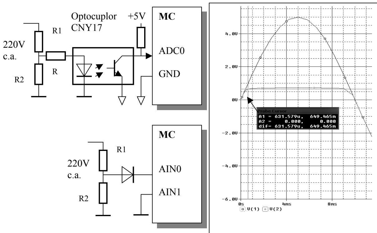
Figura 6.9: Variantă pentru schema de detectare a trecerii prin zero și simulare SPICE
