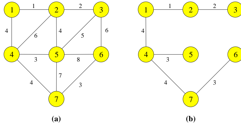
Figura 6.4 Un graf si arborele sau partial de cost minim.
