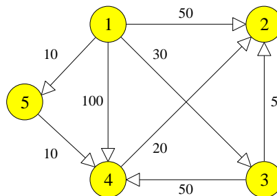
Figura 6.5 Un graf orientat.
