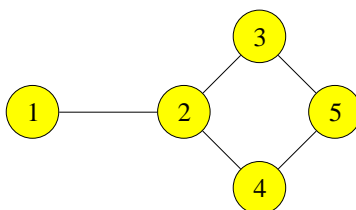
Figura 6.6 Un graf care va fi colorat.
