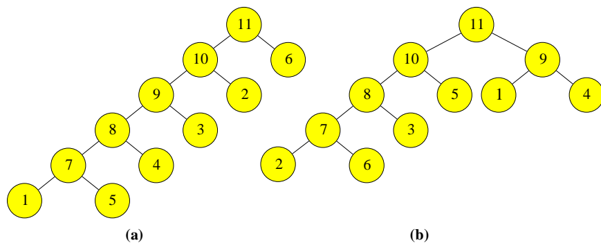
Figura 6.2 Numerotarea varfurilor arborilor din Figura 6.1.
